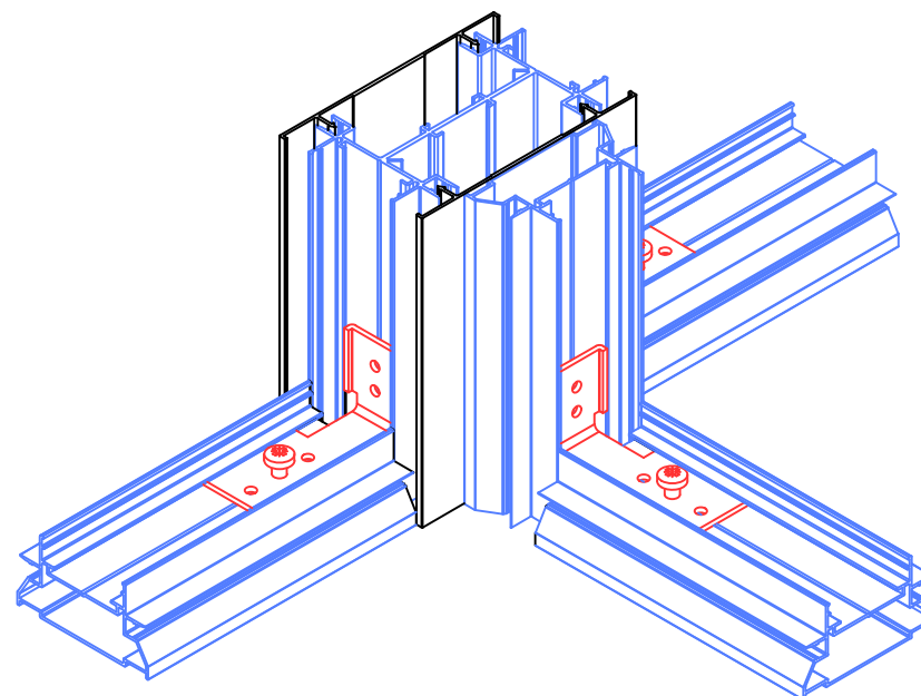
3 départs Goulotte avec couvercle d'angle
